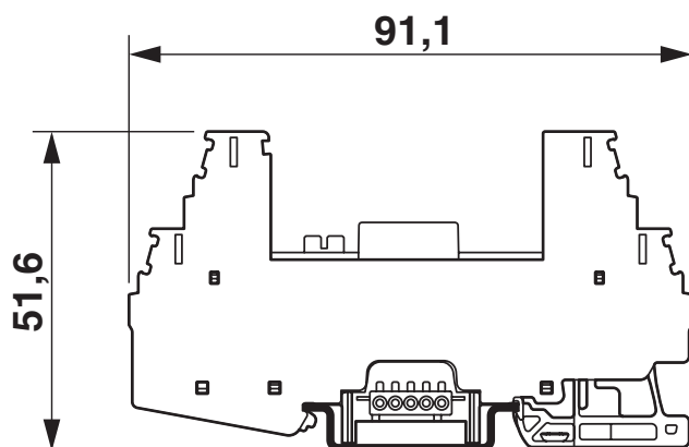
Maßzeichnung
