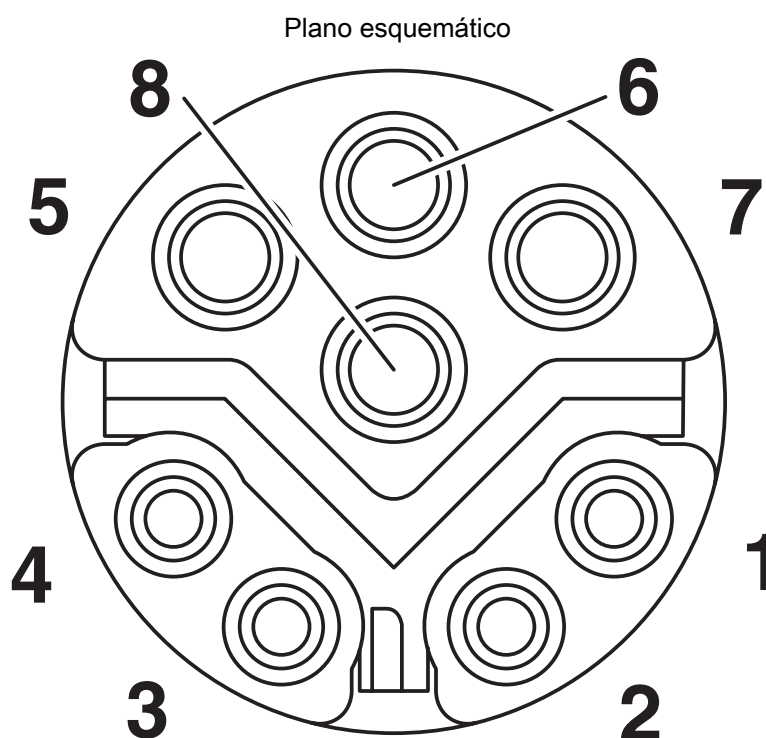
Conector hembra del esquema de polos, 8 polos, codificación Y, vista del lado del conector hembra
