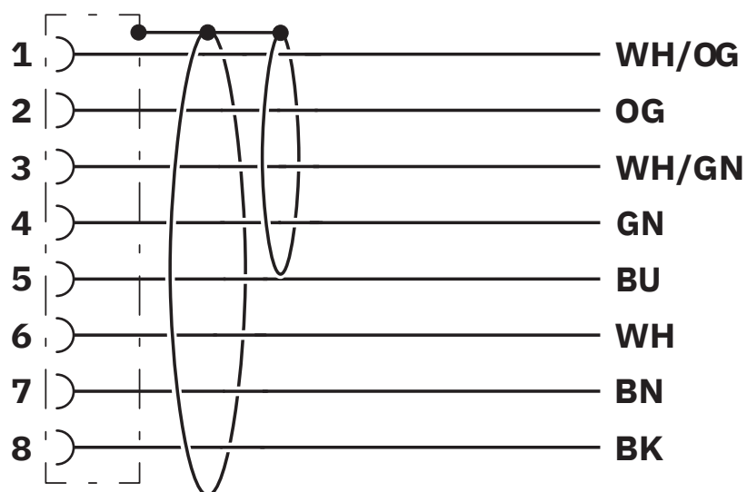
Diagrama eléctrico
