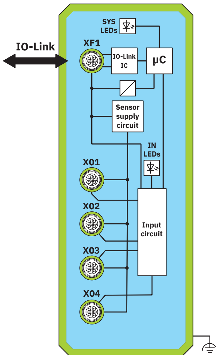
Schéma fonctionnel
