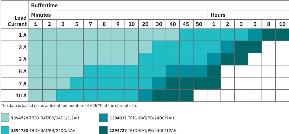
Durée d'autonomie TRIO DC UPS pour modules de batteries TRIO
