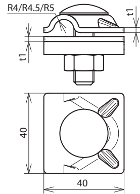
Maßbild MVK 10 FRM10X45 V4A
