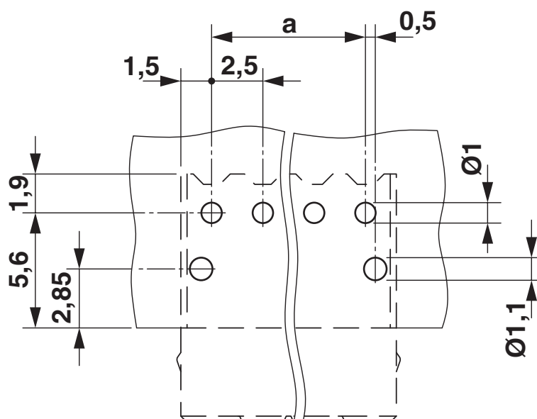
Bohrplan/Lötpadgeometrie
