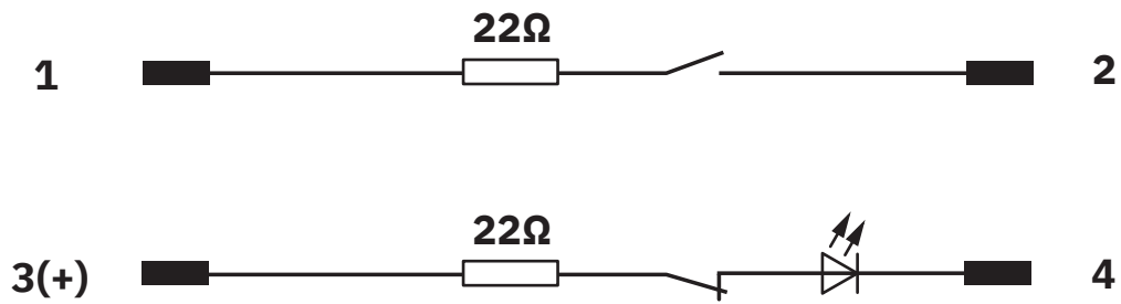
Schaltplan
