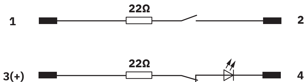
Diagrama eléctrico
