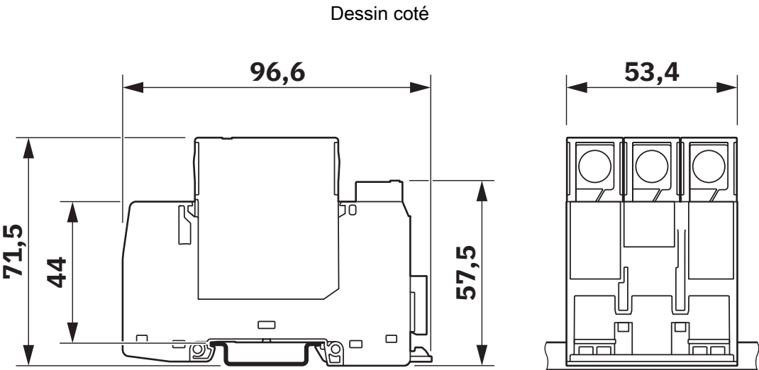
Dessin schématique
