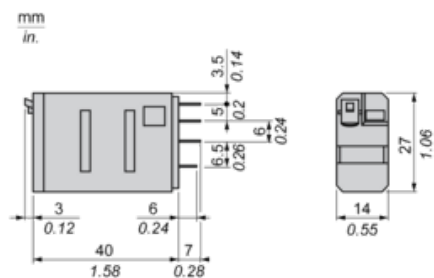
Stecker-Seitenansicht
