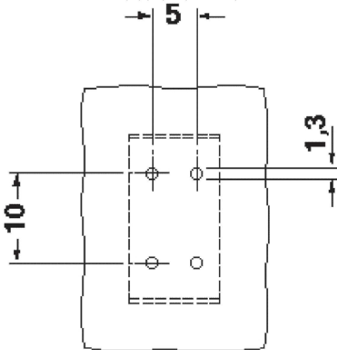
Gabarit perçage / géom. pastille soudage
