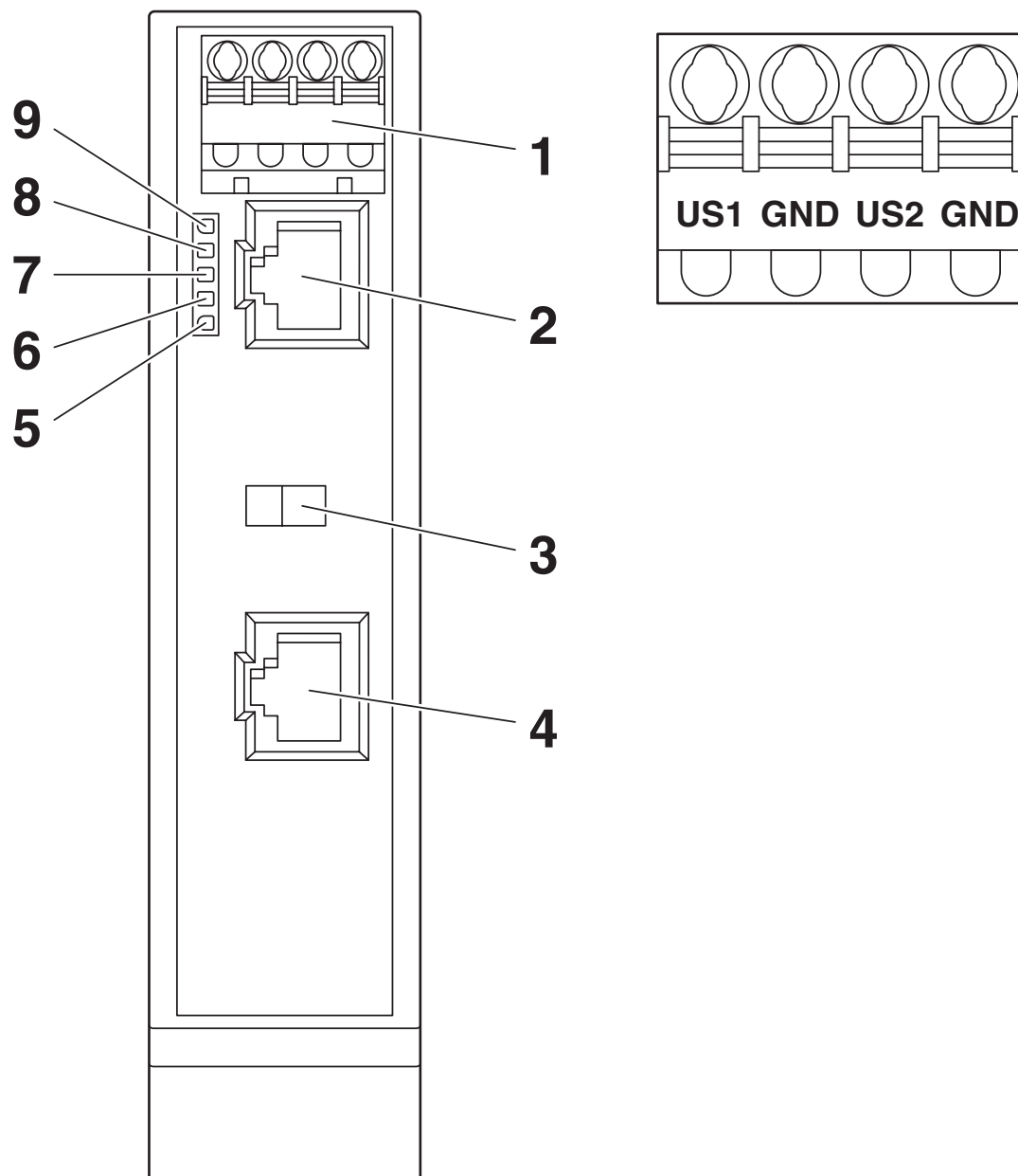
Dessin schématique
