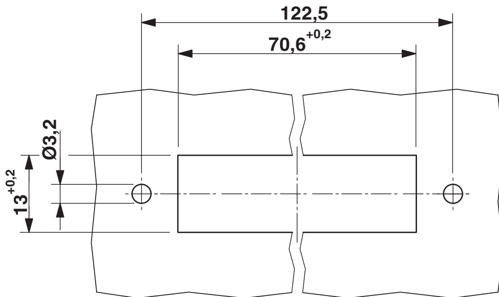
Maßzeichnung
