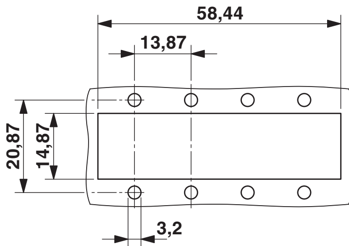
Dessin coté
