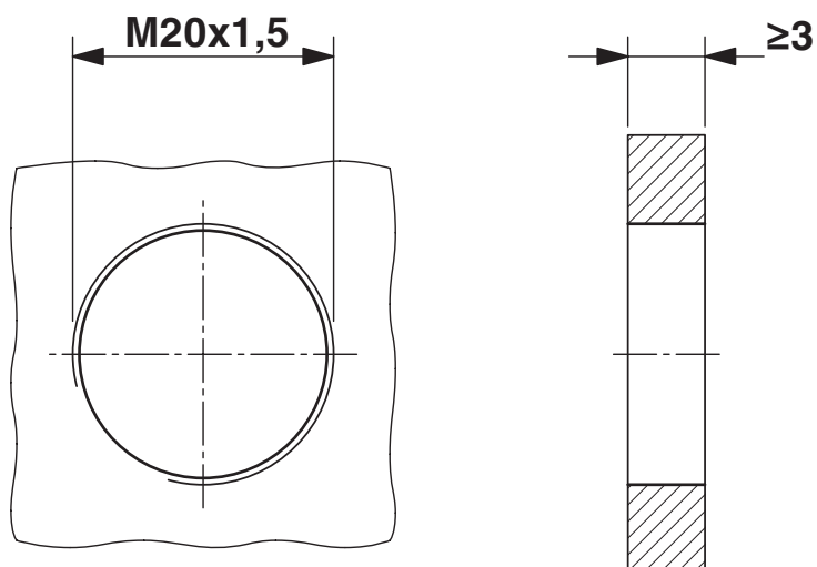
Esquema de dimensiones
