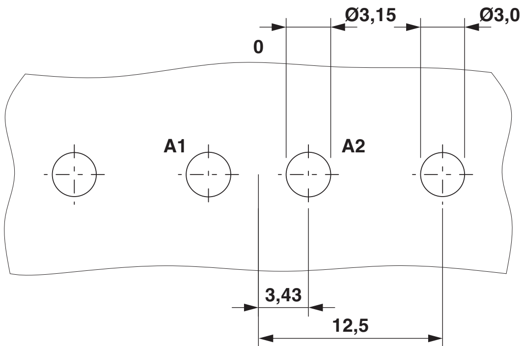
Bohrplan/Lötpadgeometrie
