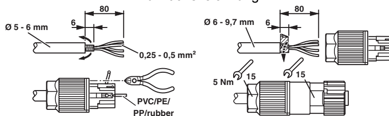
Funktionszeichnung
