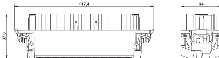
Maßzeichnung
