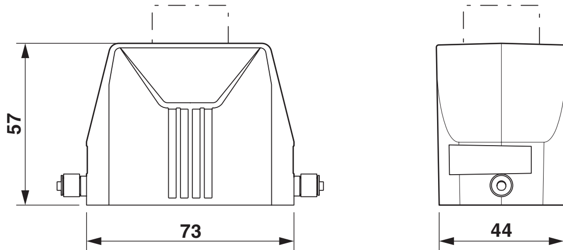
Maßzeichnung
