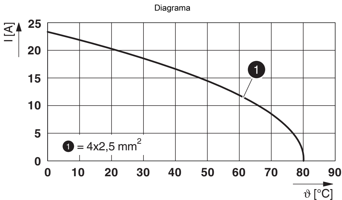
Diagrama eléctrico
