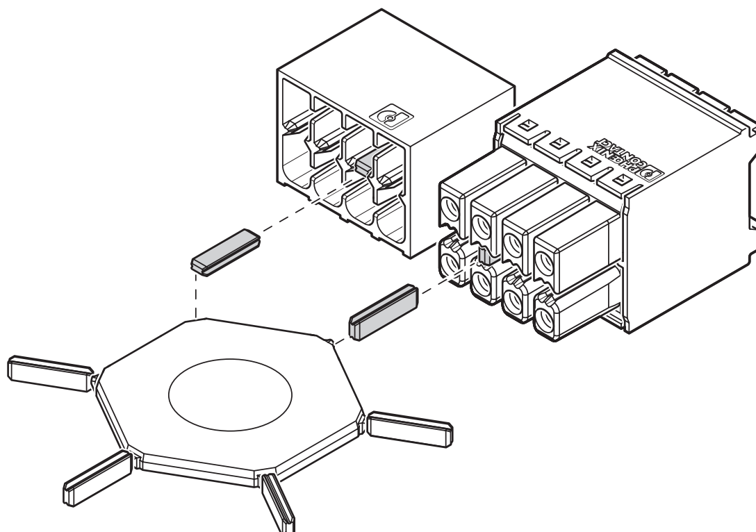
Utilisation de la languette de détournement CP-DMC...
