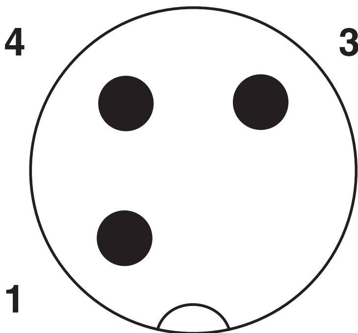
Schemazeichnung
