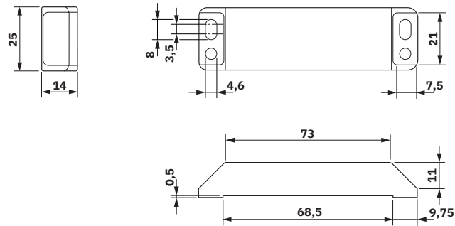
Esquema de dimensiones
