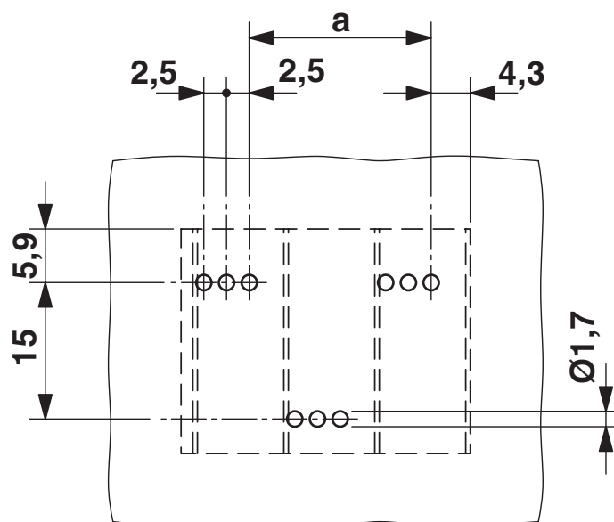
Bohrplan/Lötpadgeometrie
