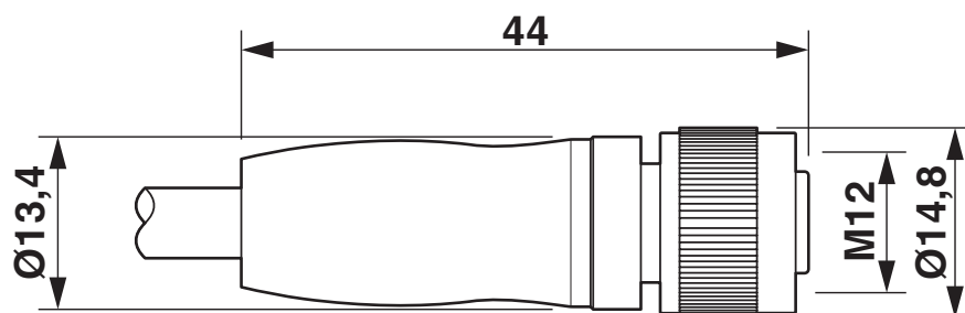
Dessin coté
