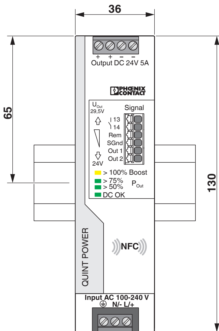
Dessin coté
