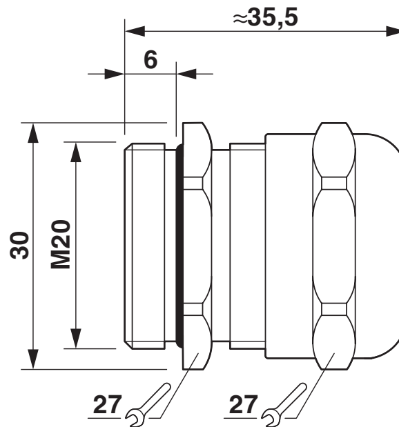
Maßzeichnung
