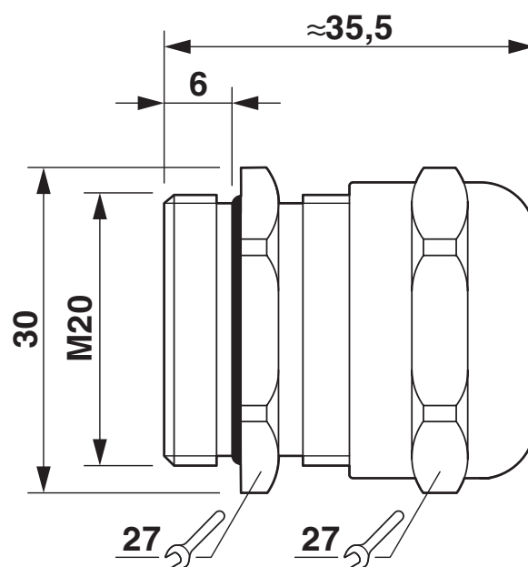
Dessin coté
