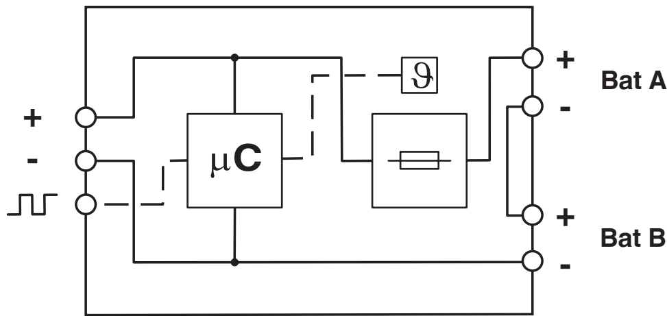
Schéma fonctionnel
