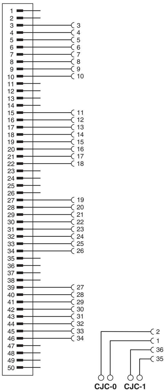
Schéma de connexion
