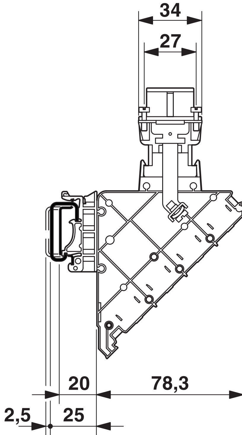
Dessin coté
