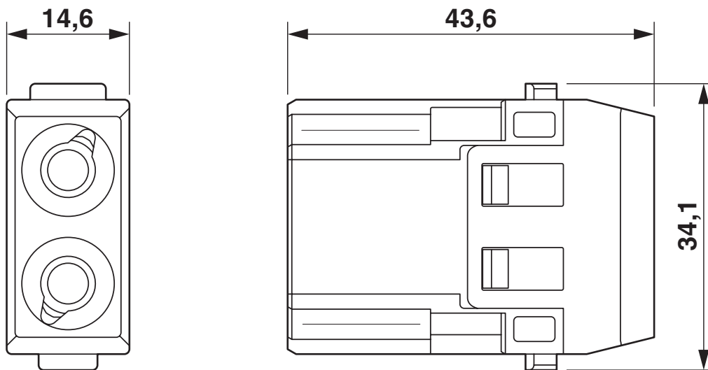
Maßzeichnung
