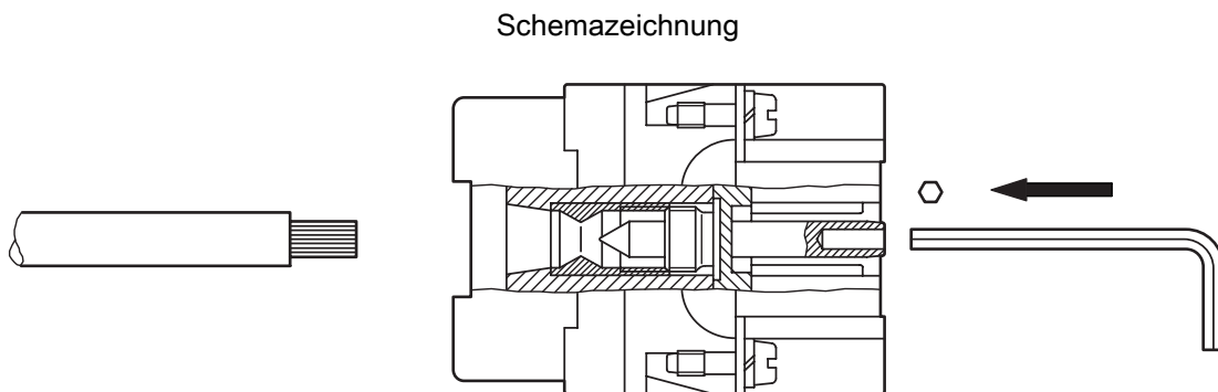
Axialanschluss (2 mm Innensechskantschlüssel)
