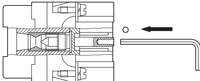
Plano esquemático
