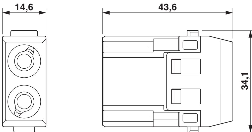
Dessin coté
