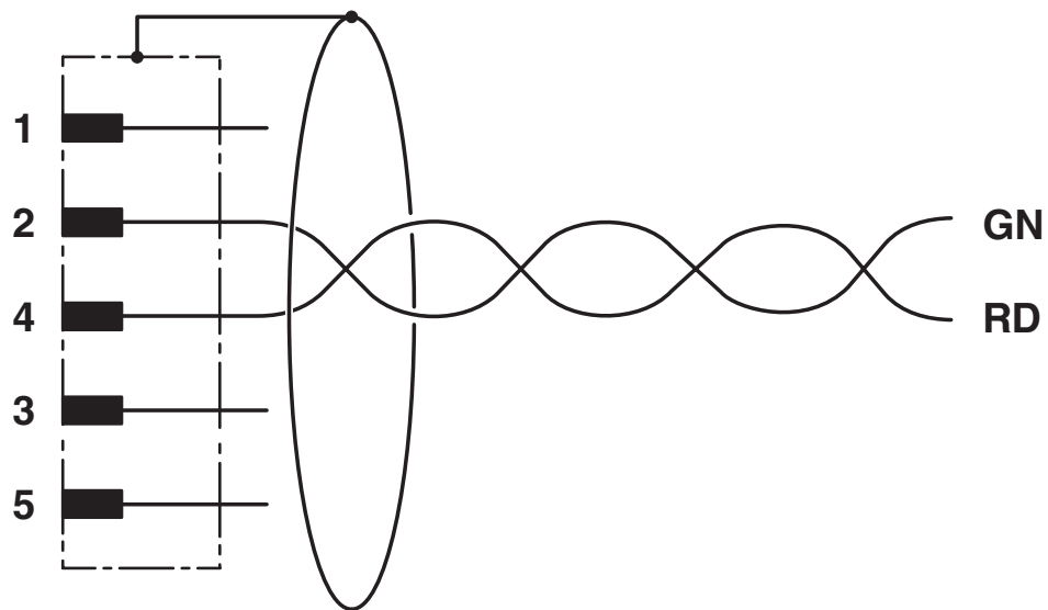
Schaltplan
