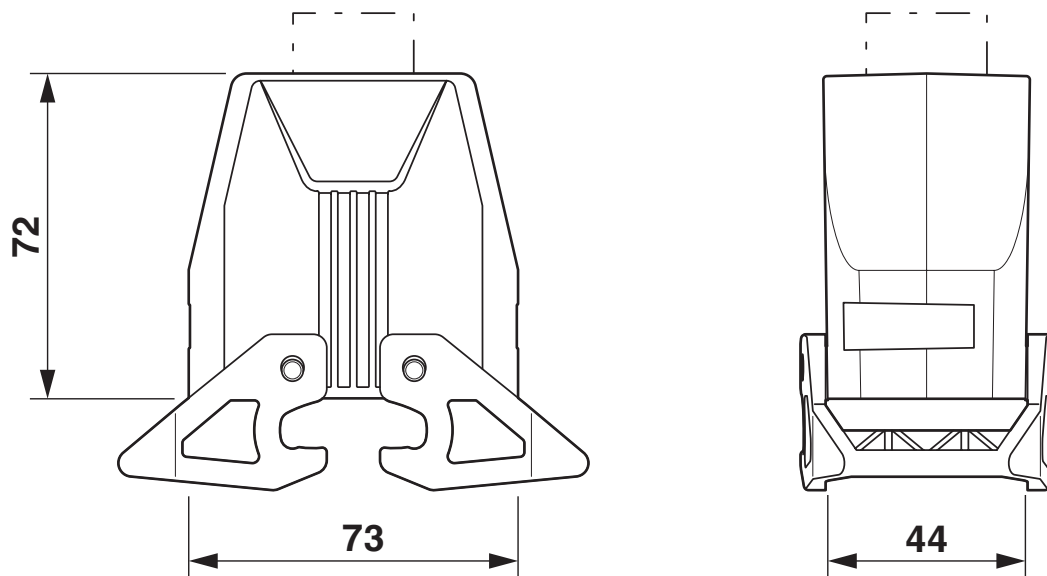
Maßzeichnung
