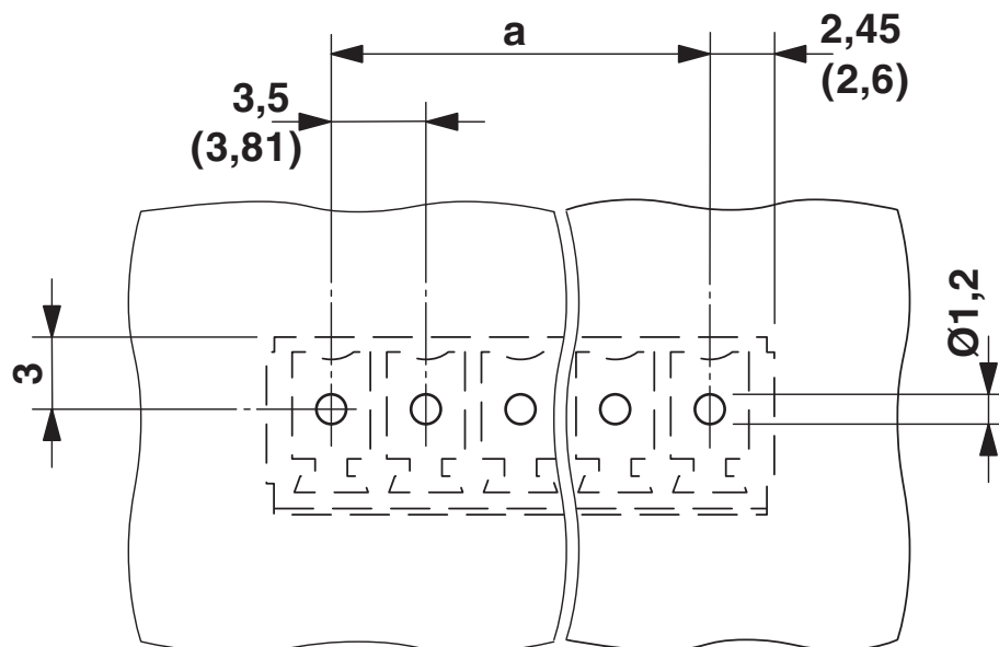
Bohrplan/Lötpadgeometrie
