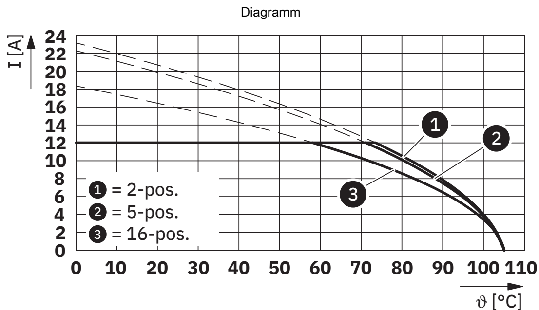
Typ: FKCN 2,5/...-STF mit DFK-MSTB 2,5/...-GF
