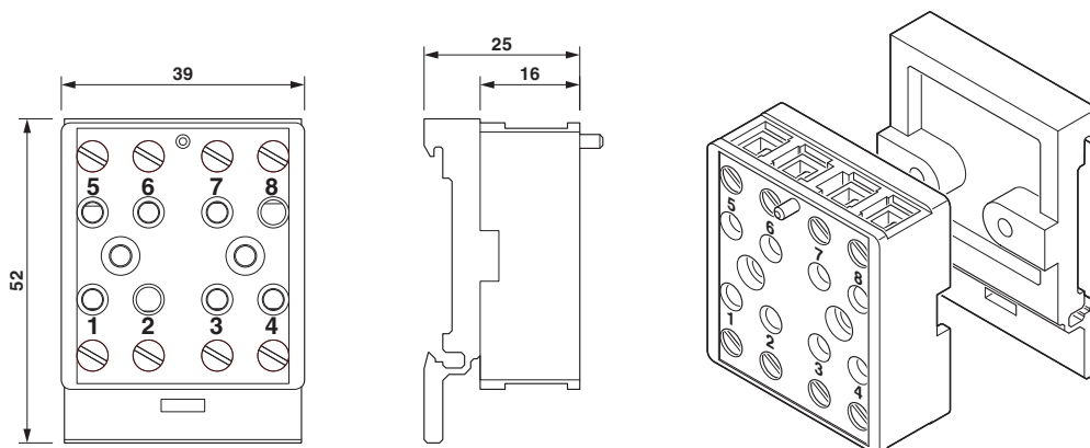
Dessin coté
