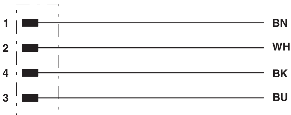
Diagrama eléctrico
