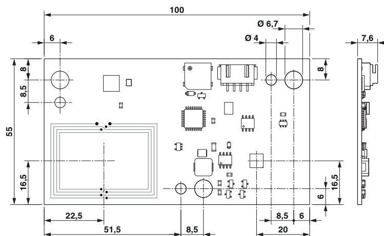
Dessin coté
