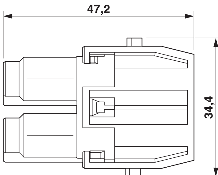
Dessin coté
