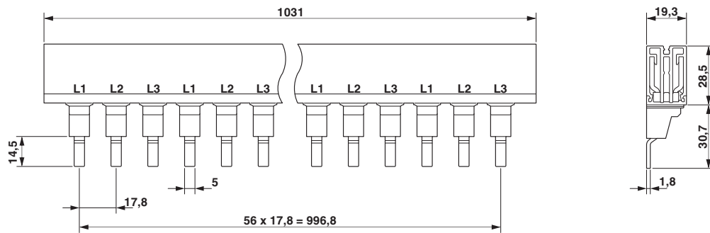
Maßzeichnung
