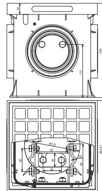
Maßbild UFTSK 7.10 FL40 197X197X204 K
