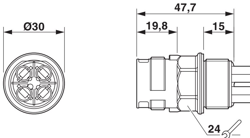
Esquema de dimensiones
