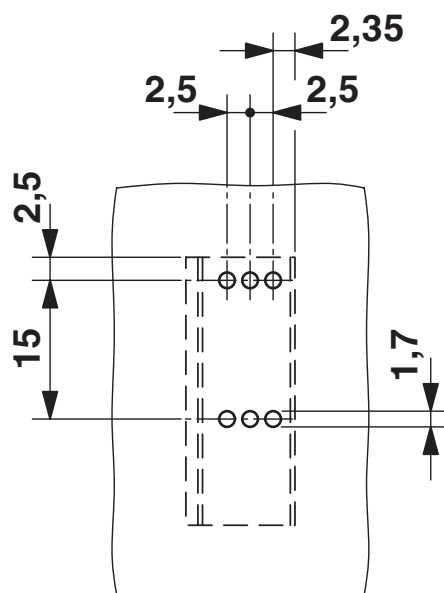
Bohrplan/Lötpadgeometrie
