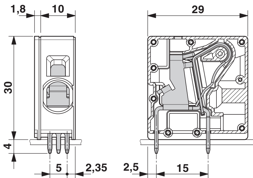
Maßzeichnung
