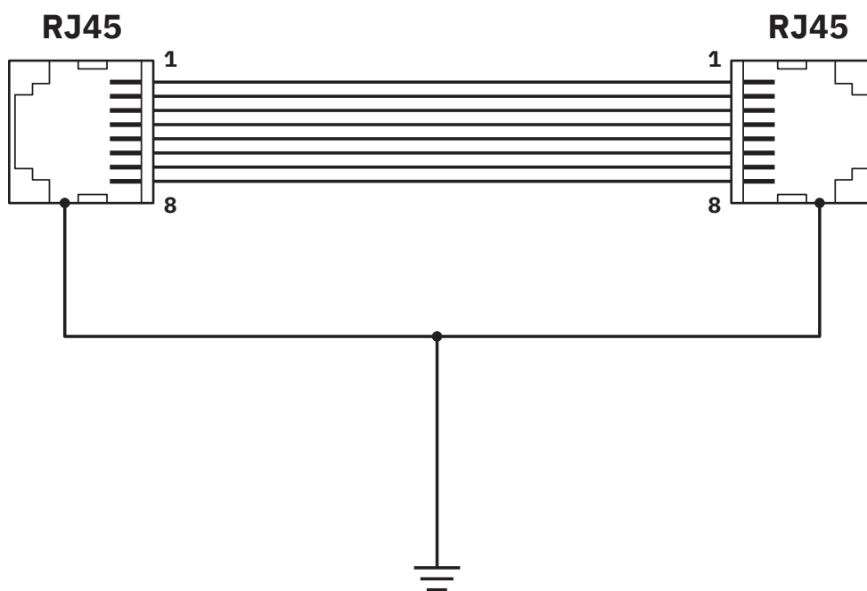
Diagrama eléctrico
