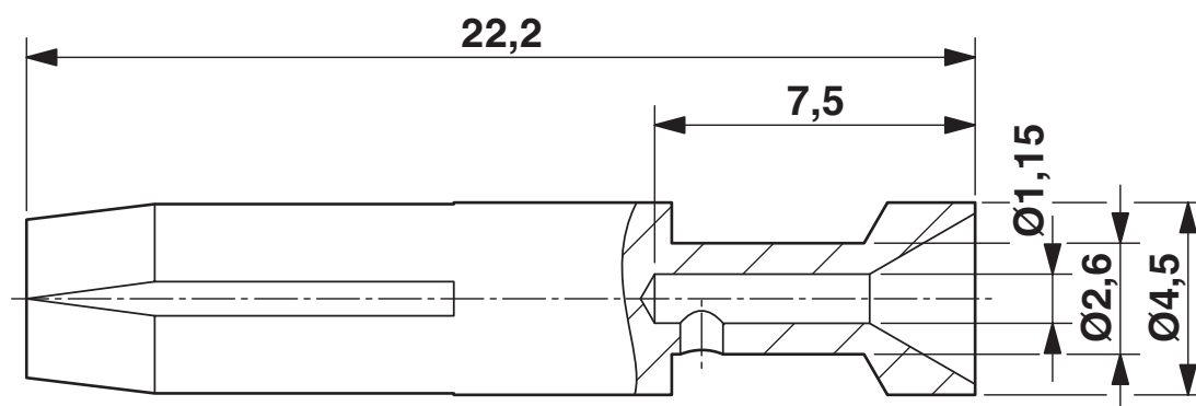
Dessin coté
