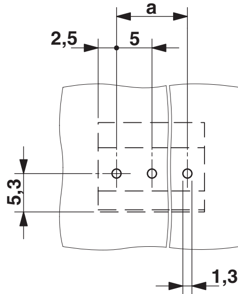
Bohrplan/Lötpadgeometrie
