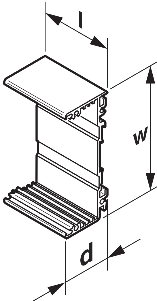
Dessin coté
